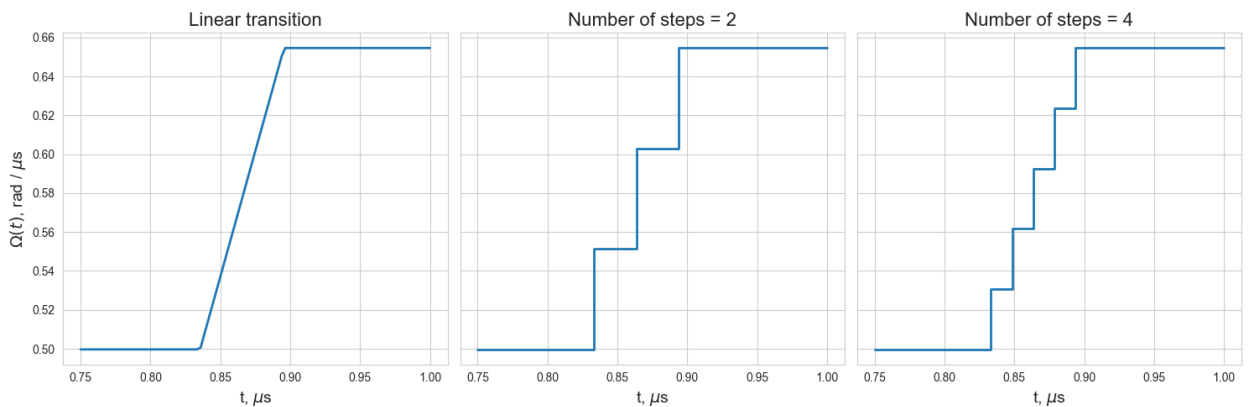
Рис. 2: Пример кусочно-постоянной равномерной аппроксимации одного линейного перехода частоты Раби с использованием двух и четырёх шагов.
