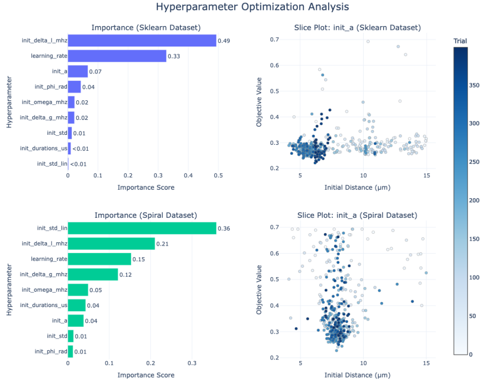
Рис. 6: Сравнительный анализ оптимизации гиперпараметров для многомерного (верхний ряд) и спирального (нижний ряд) датасетов.
