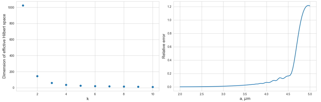
Рис. 4: Графический анализ ридберговской блокады. Слева: Зависимость размерности гильбертова пространства разрешённых состояний от числа заблокированных атомов k для цепочки из 10 атомов. Размерность полного пространства 2^{10} = 1024 . Справа: Зависимость относительной ошибки аппроксимации ридберговской блокады от расстояния между атомами для системы из 3 атомов. Эффективный радиус блокады R_b соответствует началу экспоненциального роста ошибки и в данном случае равен 4.5 \mu m .
