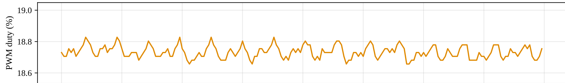
D3: Kp 1.0, \alpha 0.5 → PWM jitter 0.034 % (-69 %)
