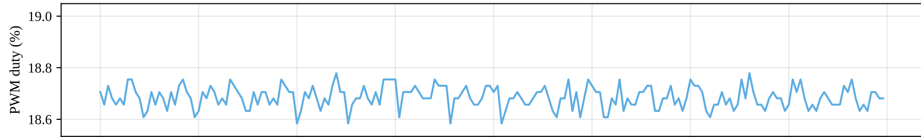
F2: Kp 0.8, Ki 25.0 → PWM jitter 0.054 % (-51 %)
