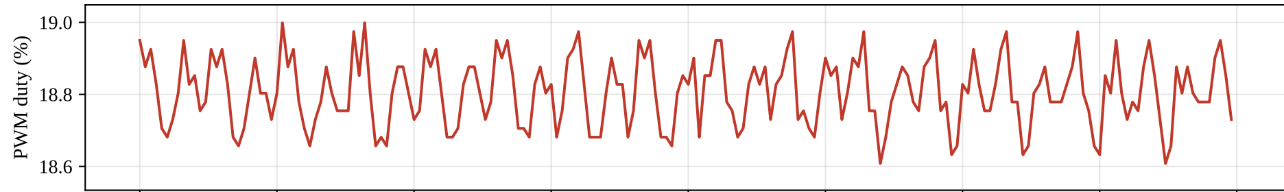
A: baseline (Kp 1.56, Ki 41.2) → PWM jitter 0.109 %
