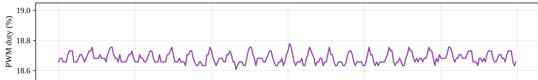
F1: Kp 0.8, \alpha 0.5 → PWM jitter 0.030 % (-73 %)
