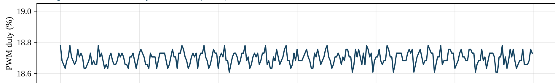
D3: Kp 1.0, \alpha 0.5 → PWM jitter 0.034 % (-69 %)
