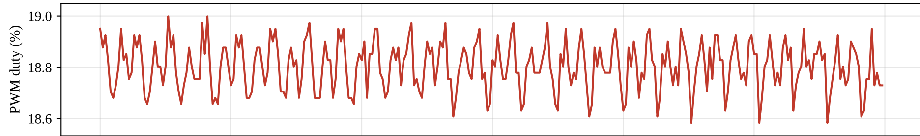
A: baseline (Kp 1.56, Ki 41.2) → PWM jitter 0.109 %
