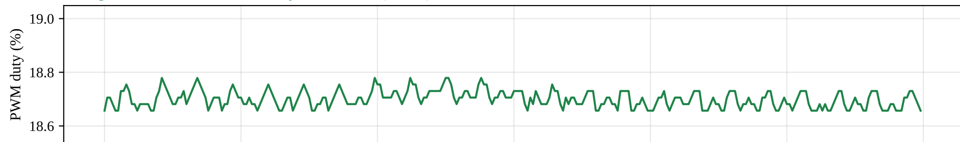
F3: Kp 0.8, Ki 25.0, \alpha 0.5 → PWM jitter 0.027 % (-76 %)
