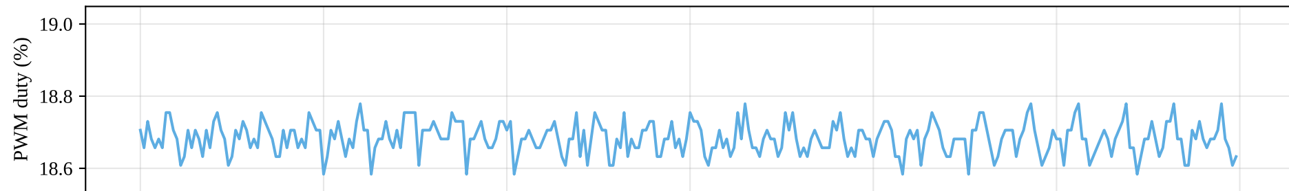
F4: Kp 0.8, Ki 15.0 → PWM jitter 0.051 % (-54 %)
