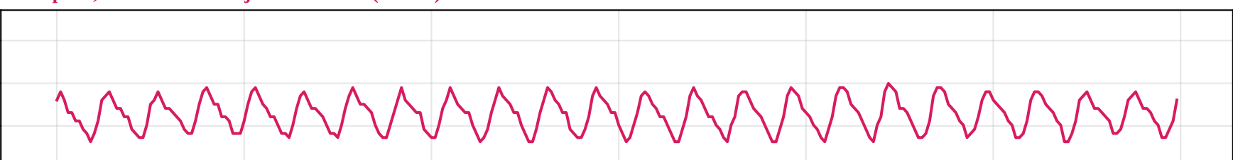
D3: Kp 1.0, \alpha 0.5 → PWM jitter 0.050 % (-61 %)
