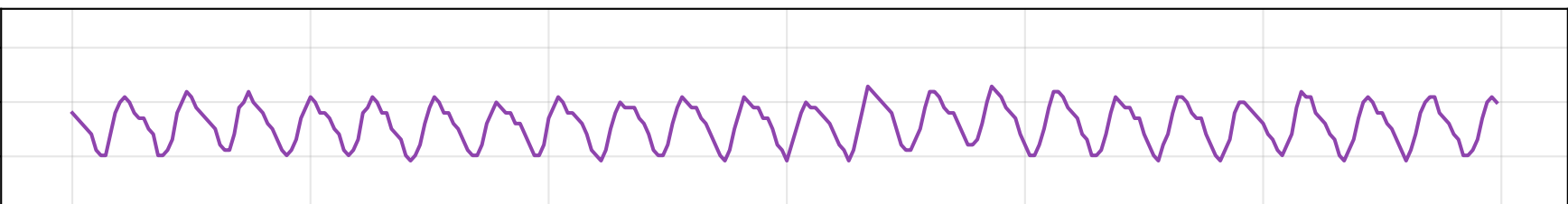
B2: \alpha 0.3 → PWM jitter 0.047 % (-63 %)
