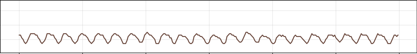
D4: Kp 1.0, α 0.3 → PWM jitter 0.031 % (-75 %)
