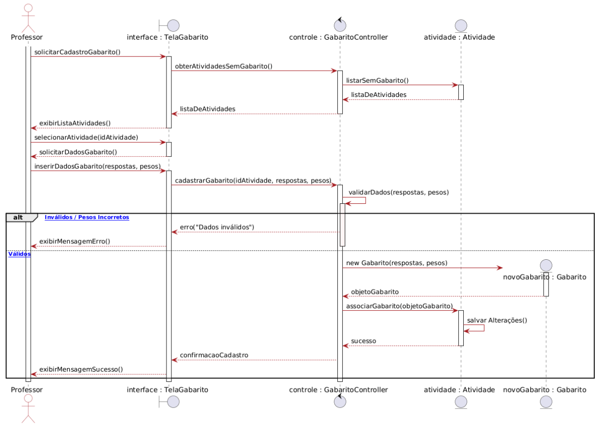
Diagrama de Sequência - UC012: Cadastrar Gabarito das Atividades
