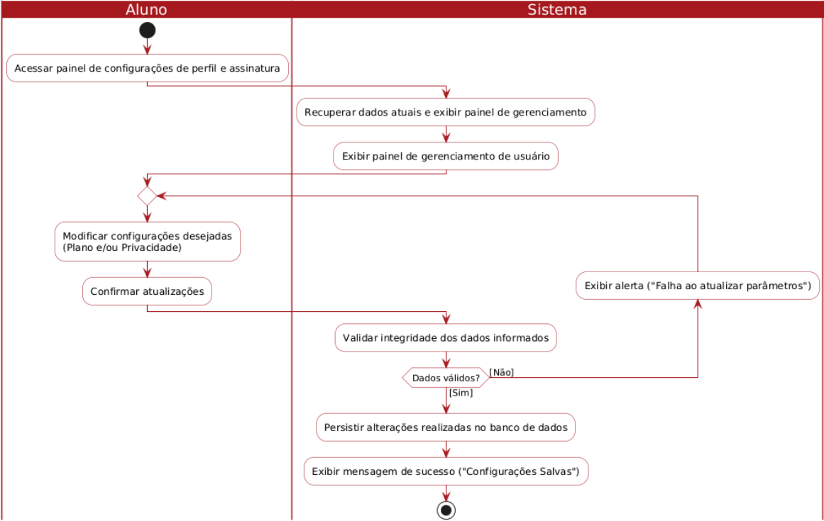
Diagrama de Atividades - UC007: Gerenciar Plano e Privacidade
