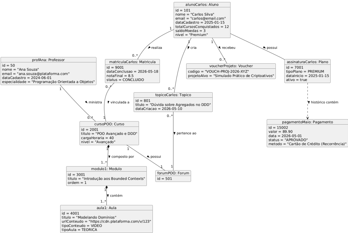
Diagrama de Objetos - Plataforma de Educação Continuada (Cenário Premium)
