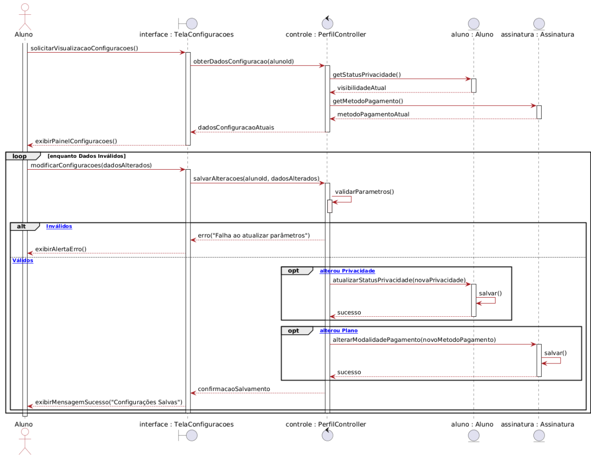
Diagrama de Sequência - UC007: Gerenciar Plano e Privacidade
