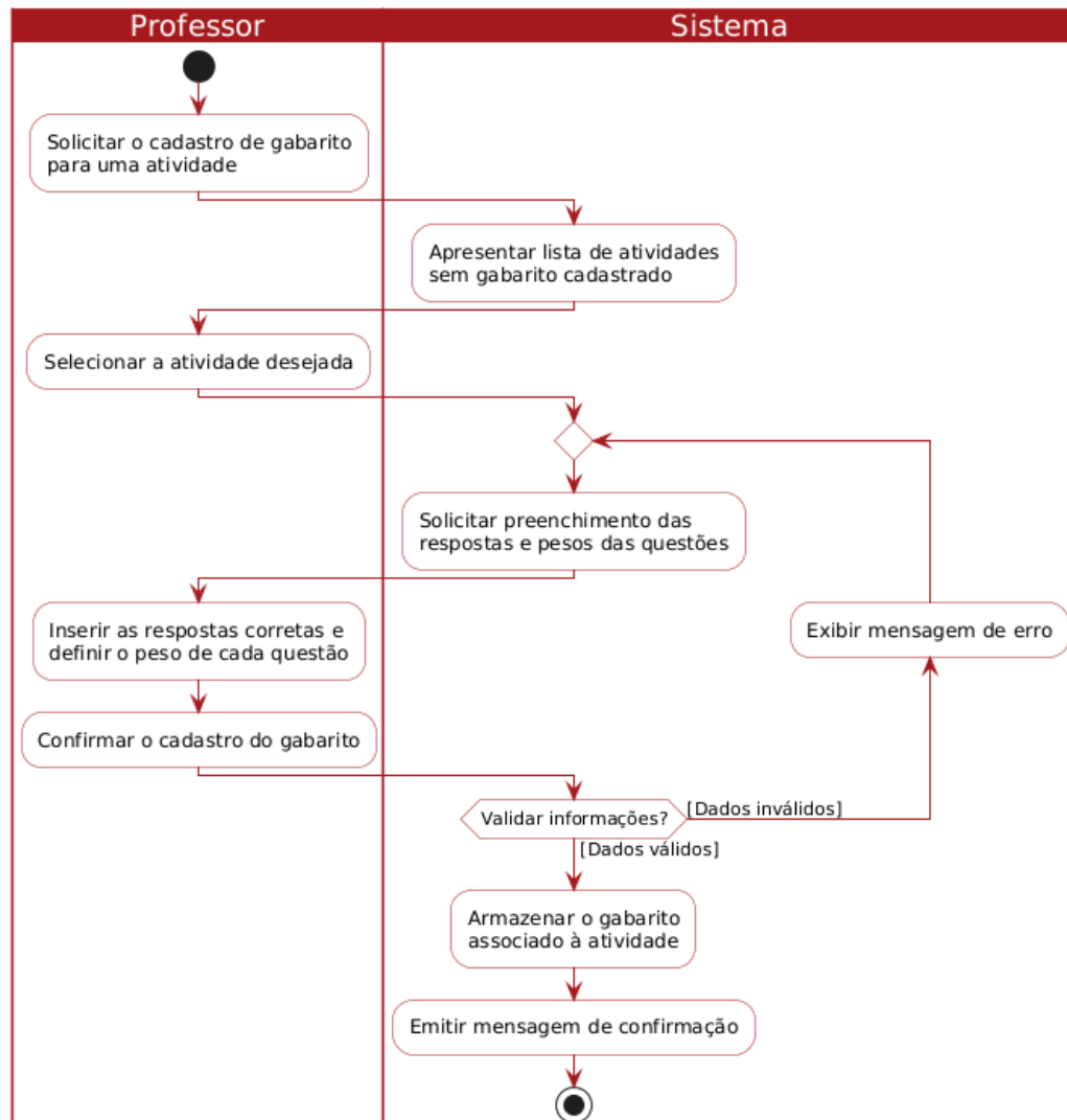
Diagrama de Atividades - UC012: Cadastrar Gabarito das Atividades
