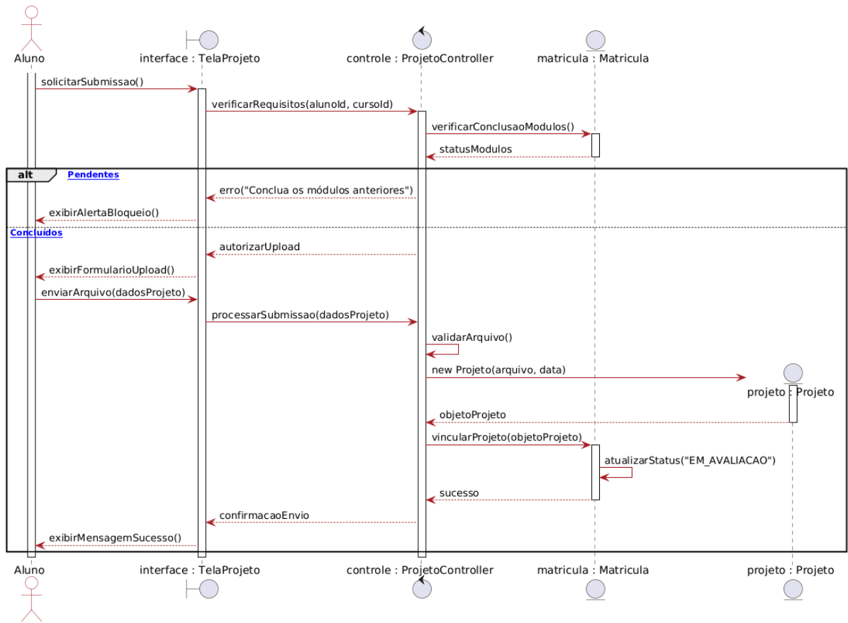
Diagrama de Sequência - UC005: Enviar Projeto Final
