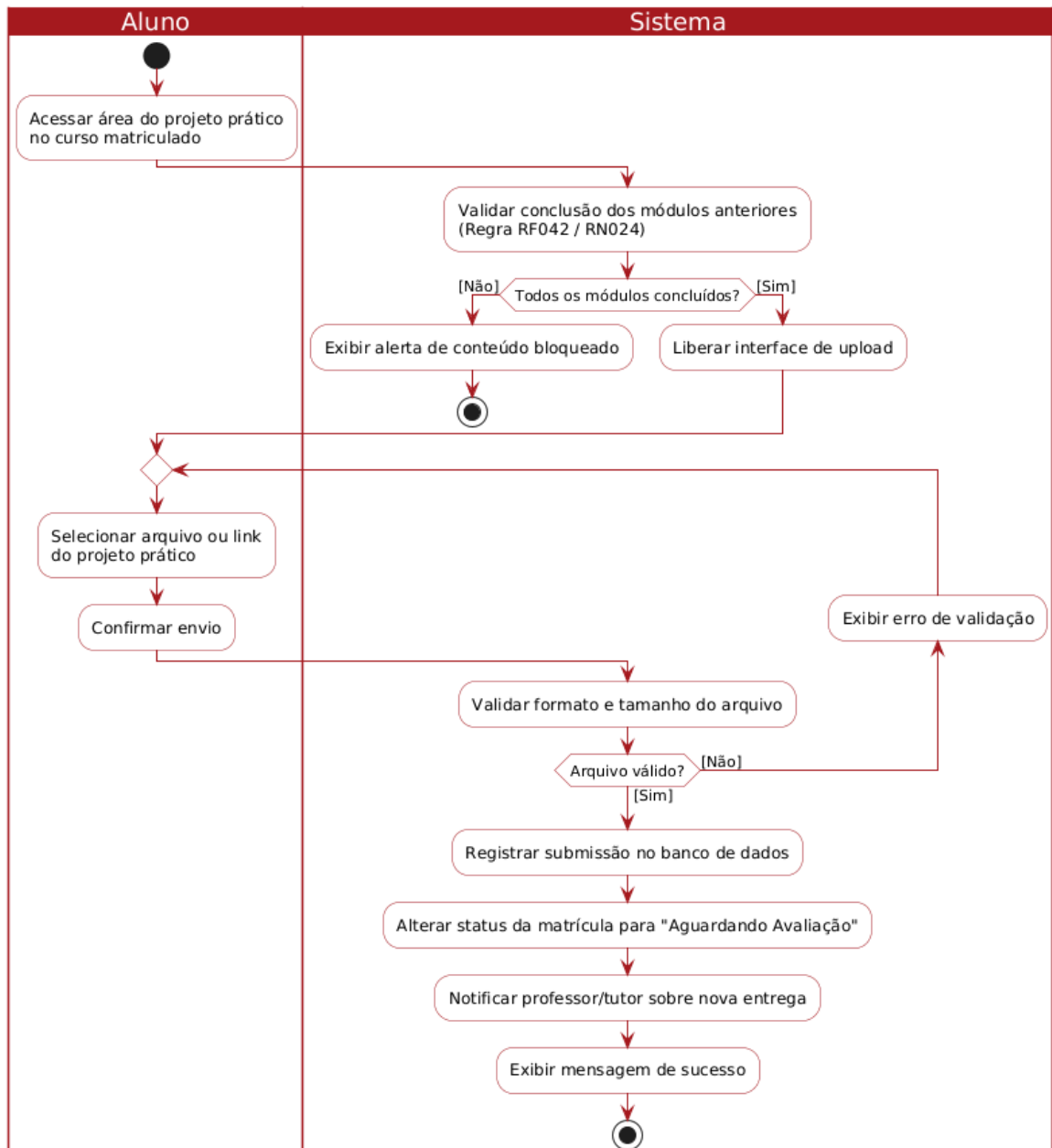
Diagrama de Atividades - UC005: Enviar Projeto Final
