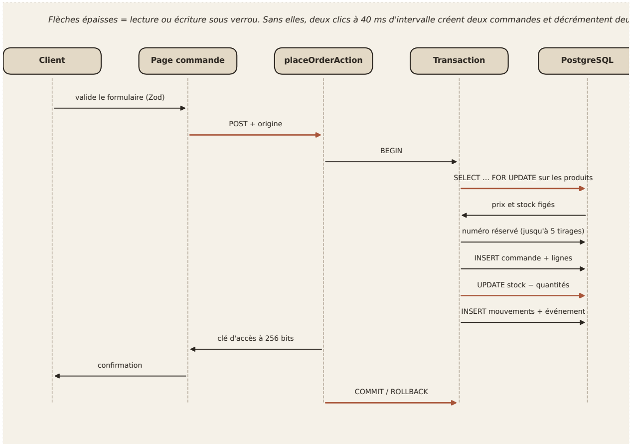
Figure 32 — Séquence : le passage de commande, minute par minute. Le diagramme le plus important du mémoire, parce que c'est là que se joue l'argent et le stock. Les quatre hachures rouges sont les quatre points où une implémentation naïve perd de la donnée. Gisement : src/actions/checkout.ts:41 · src/lib/orders.ts:67-101 .
