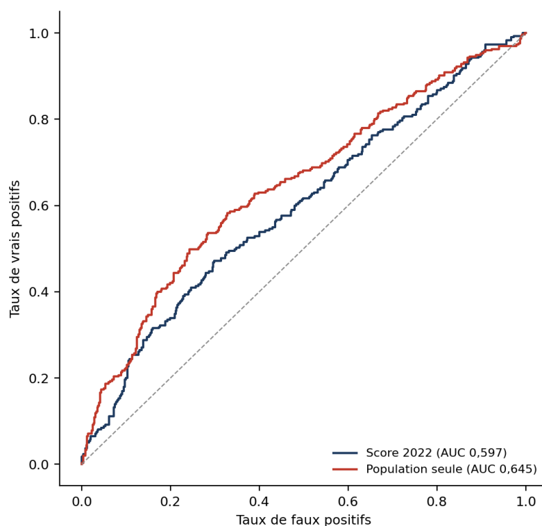
Figure 12 — Courbes ROC de la prédiction de l'équipement 2022-2026 par le score 2022 et par la population seule (cohorte, n = 777 ).
