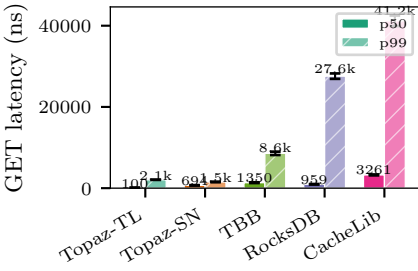
YCSB-A (64B)
