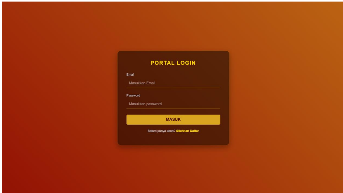
Gambar 3.10 (implementasi login)
