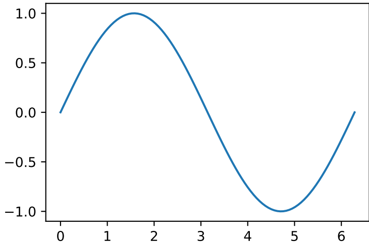
sin
