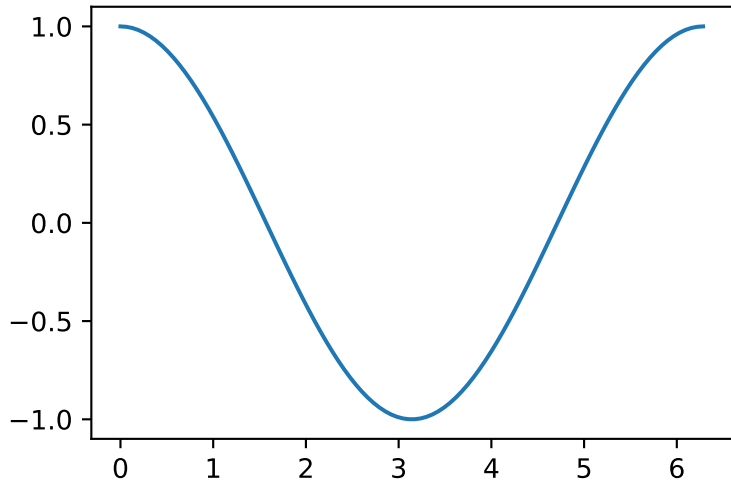
cos
