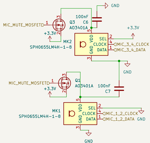
Microphones 1-2
