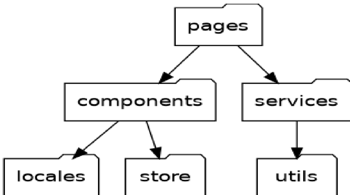
Рисунок 3 – UML діаграма пакетів web-застосунку
