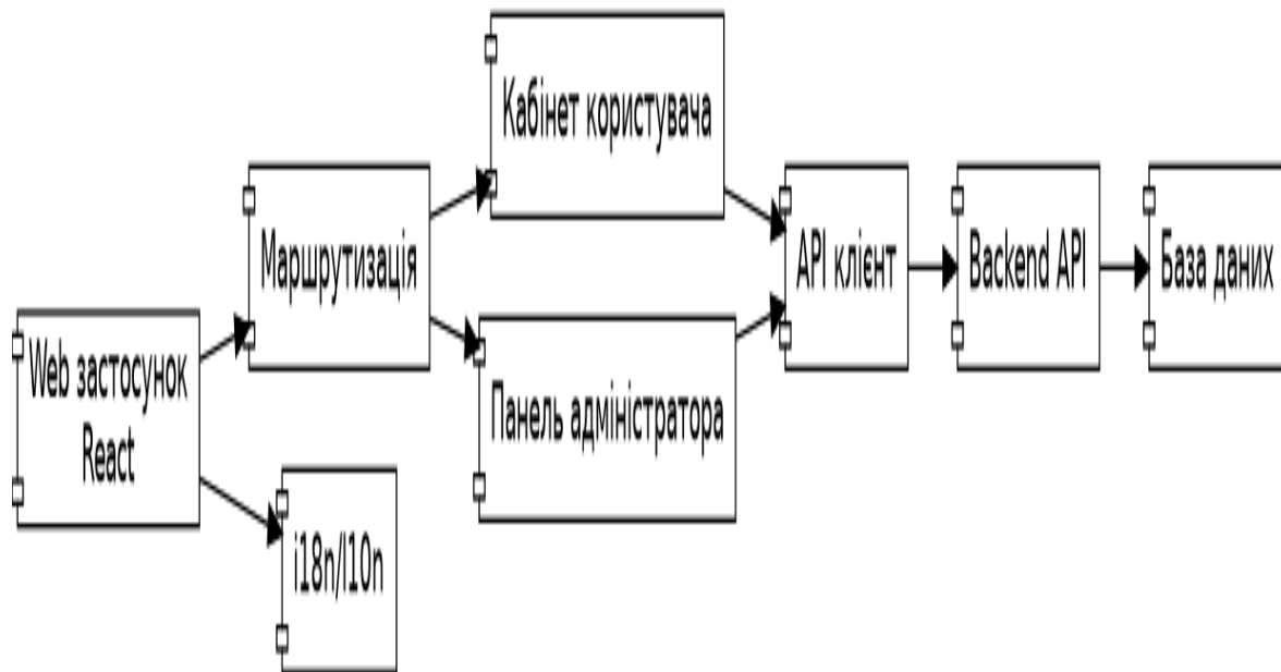
Рисунок 2 – UML діаграма компонент web-застосунку
