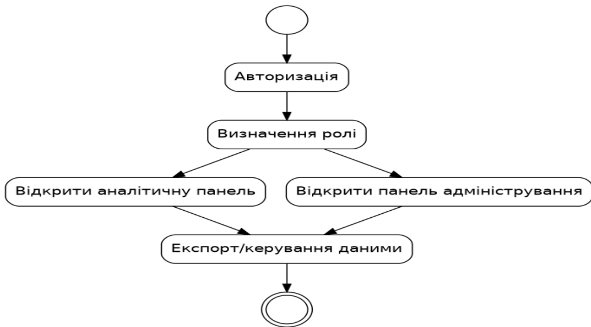
Рисунок 4 – UML діаграма діяльності користувача у web-застосунку
