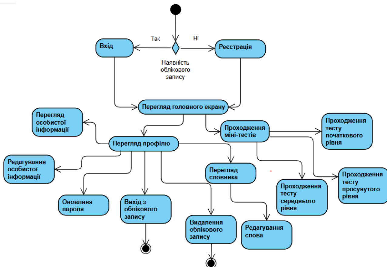
Рисунок 3.2 – Діаграма діяльності інтерактивного веб-додатку для навчання англійської мови (рисунок виконаний самостійно)
