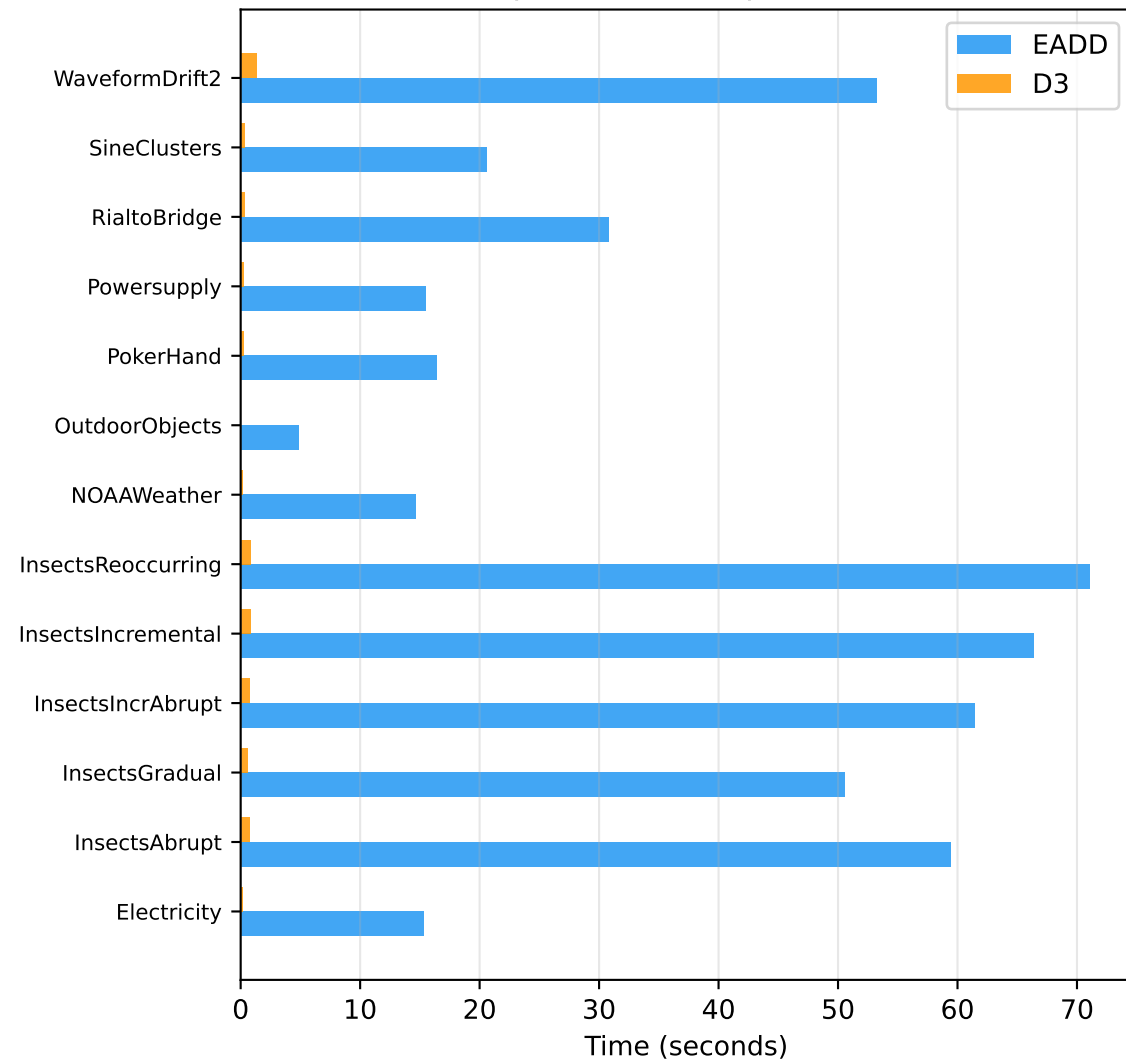
Computation Time per Dataset
