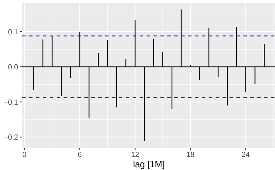
acf
