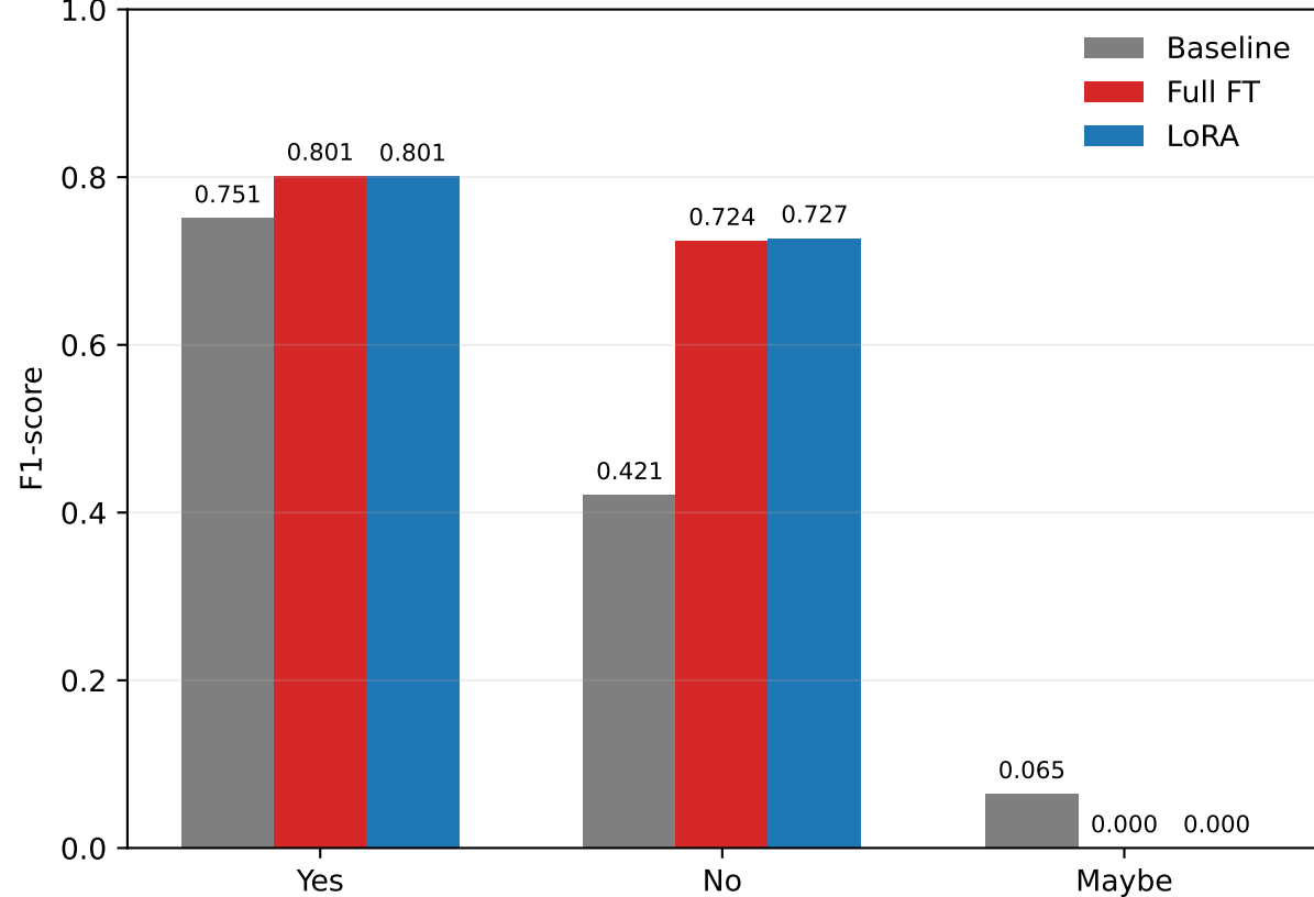
(b) Class-wise PQA-L test F1
