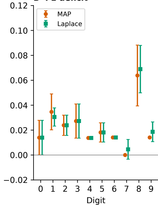
B F1 deficit
