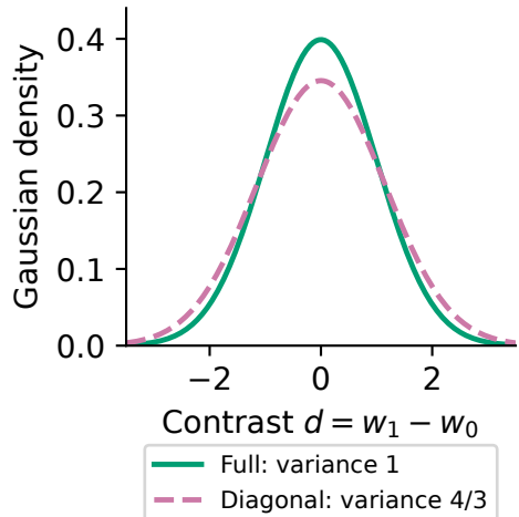
C Logit contrast
