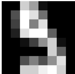
idx 792: 6 -> 4 confidence 0.57
