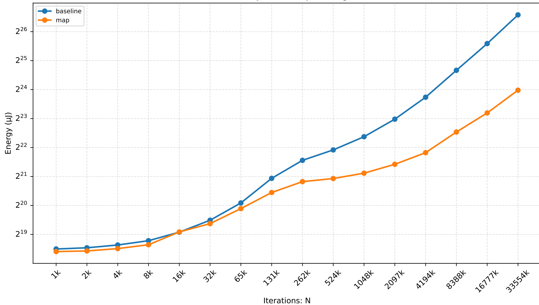
GRAALJS — lookup Scaling
