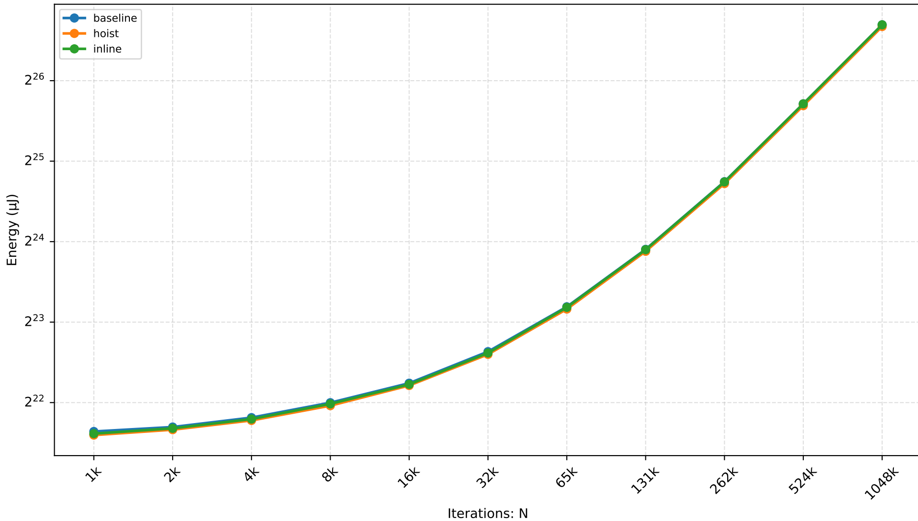
GRAALJS — loop-arr-length Scaling
