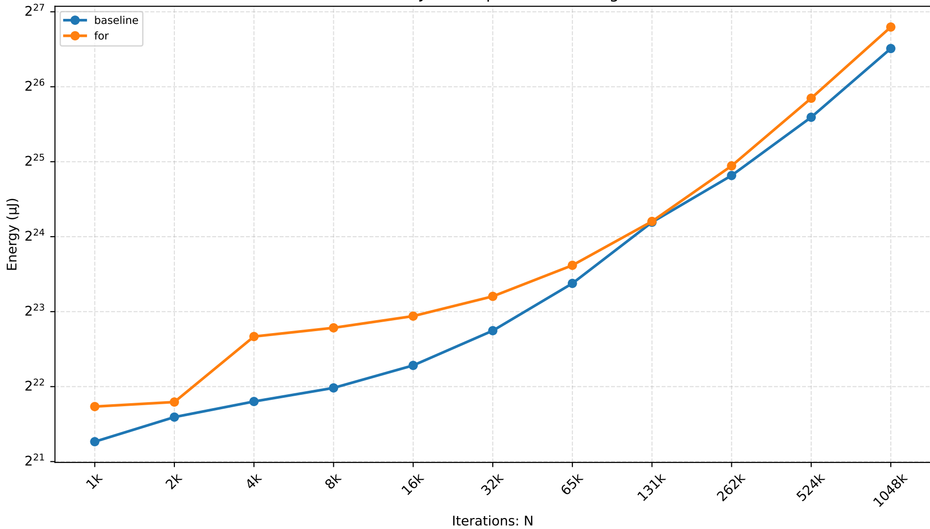
GRAALJS — map-reduce Scaling
