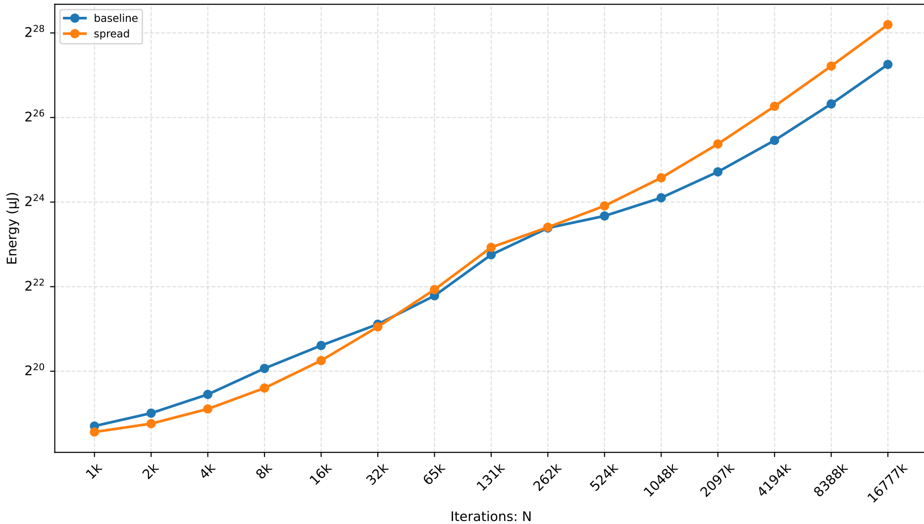
GRAALJS — object-merging Scaling
