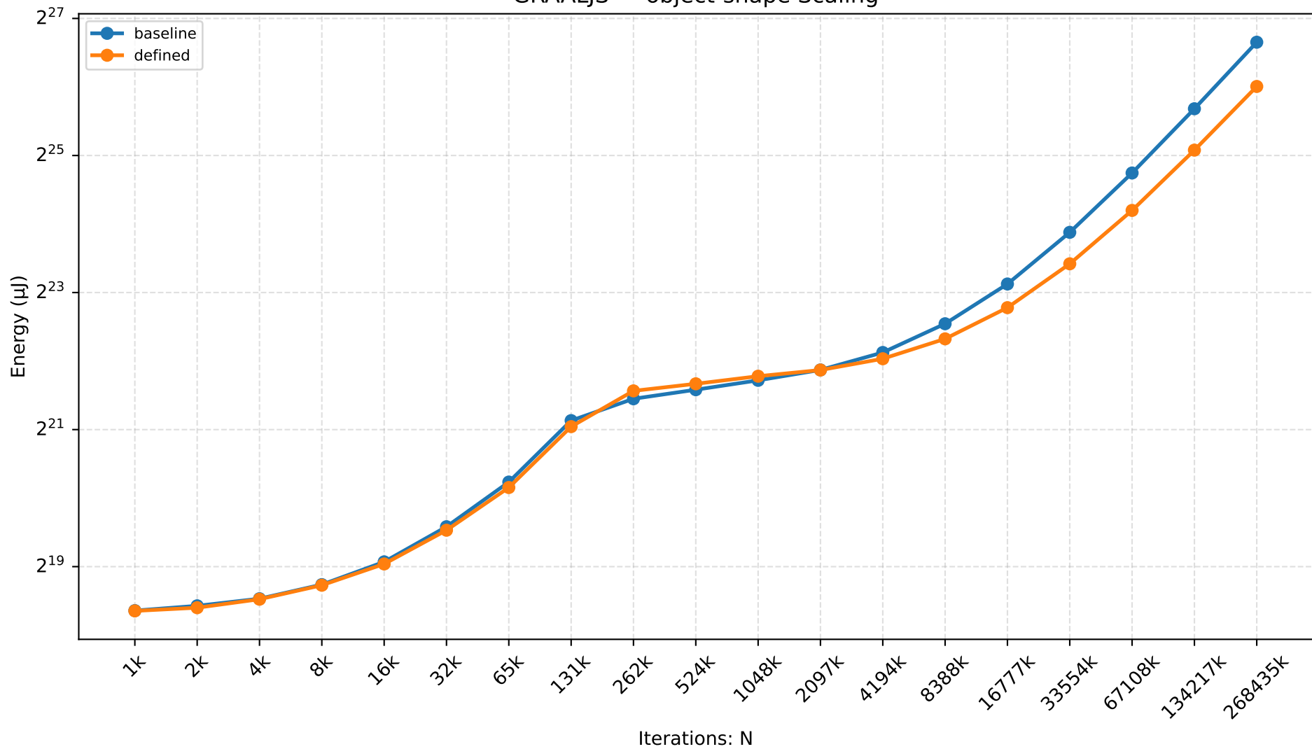
GRAALJS — object-shape Scaling
