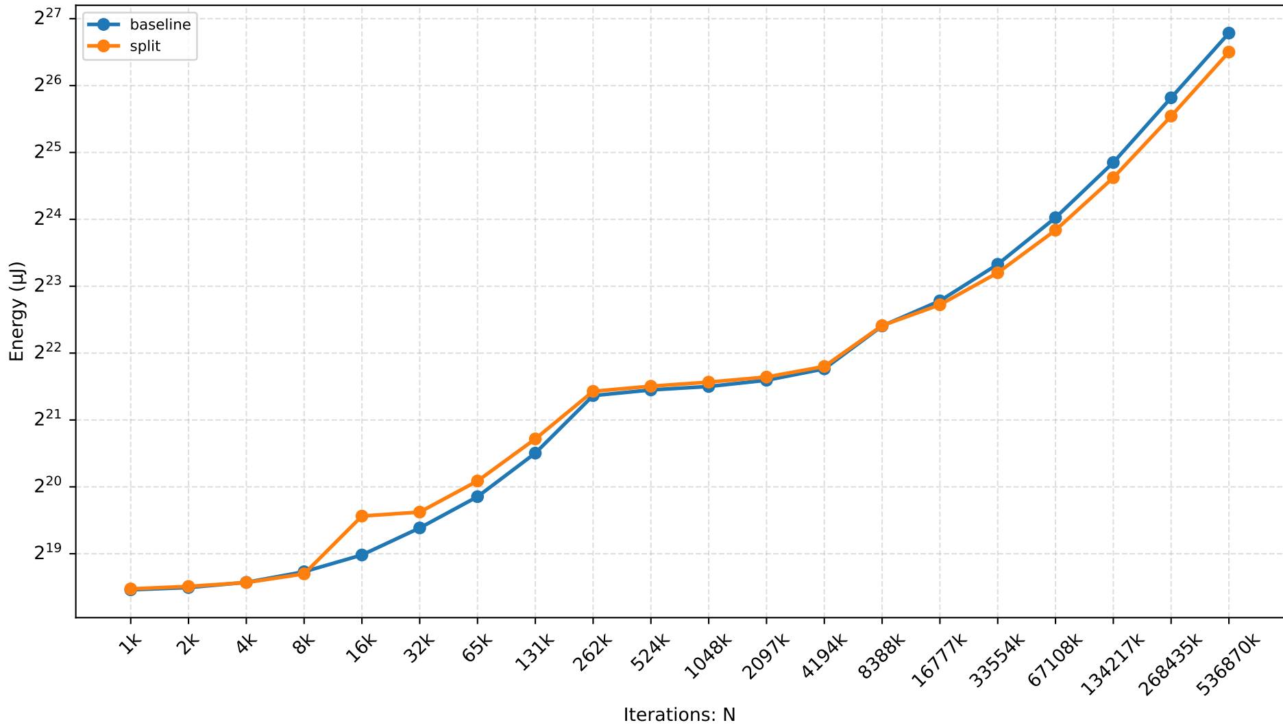
GRAALJS — polymorphic Scaling
