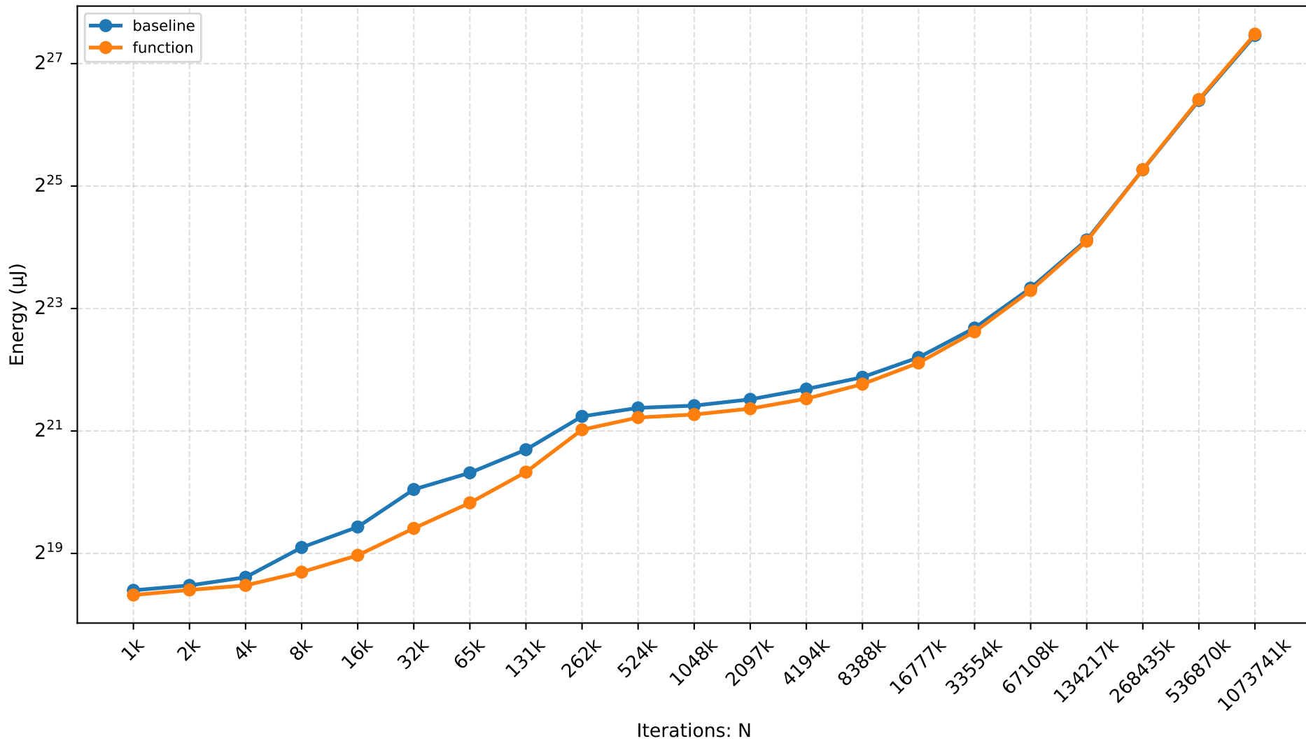
GRAALJS — prototype Scaling
