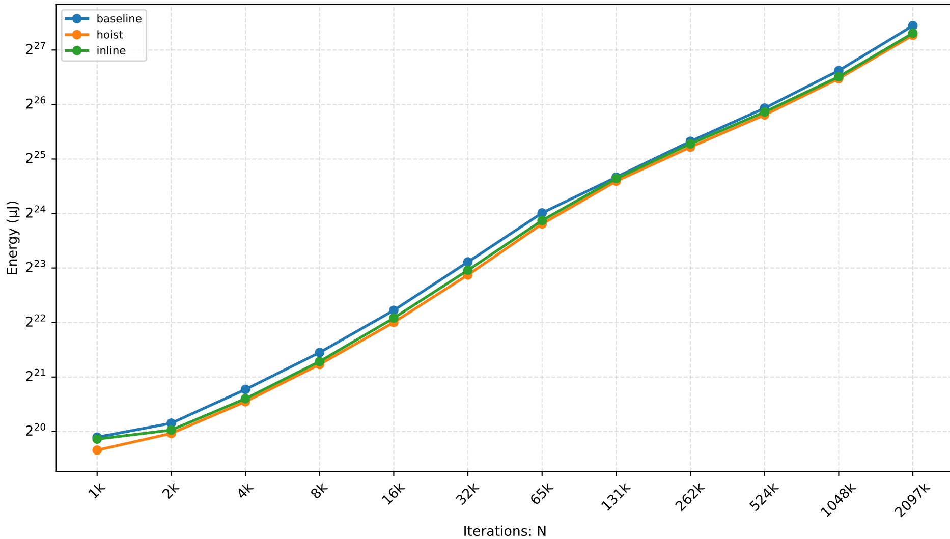
GRAALJS — regex Scaling
