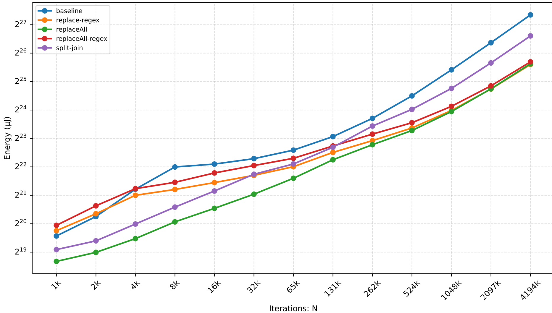
GRAALJS — replace-loop Scaling
