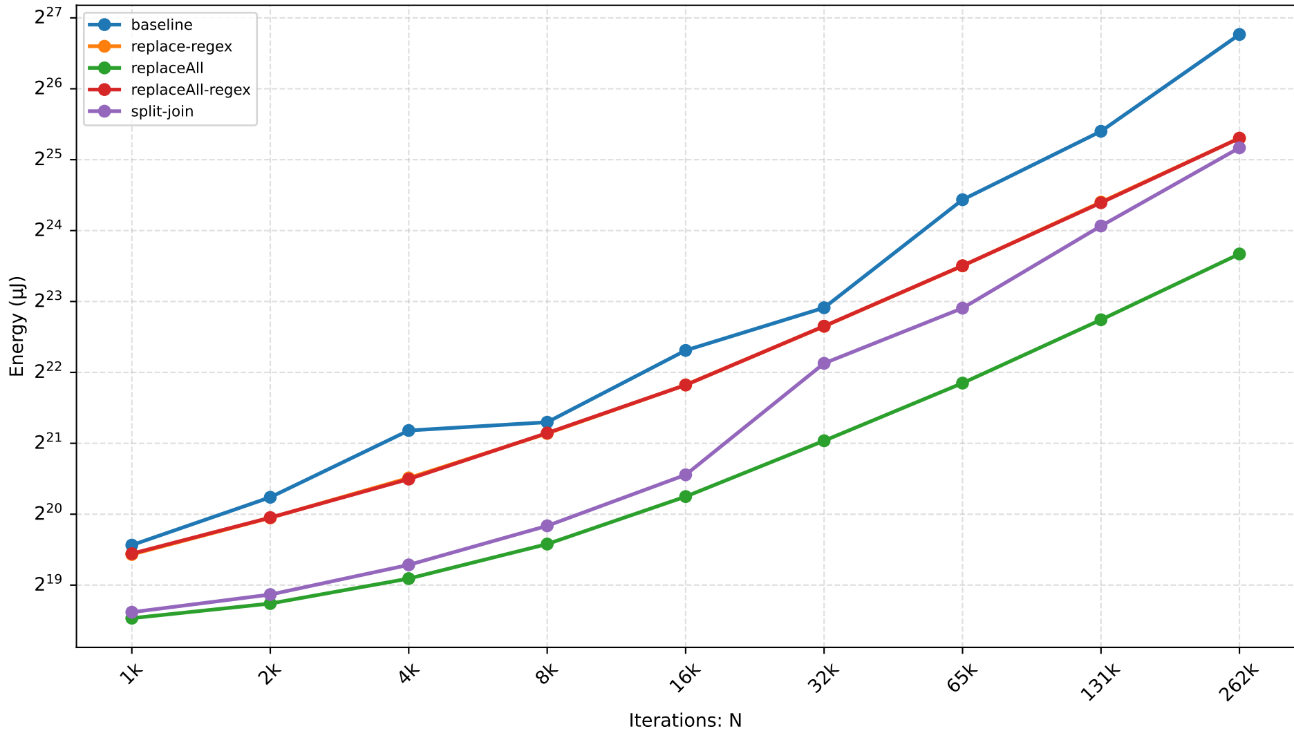
GRAALJS — replace-size Scaling
