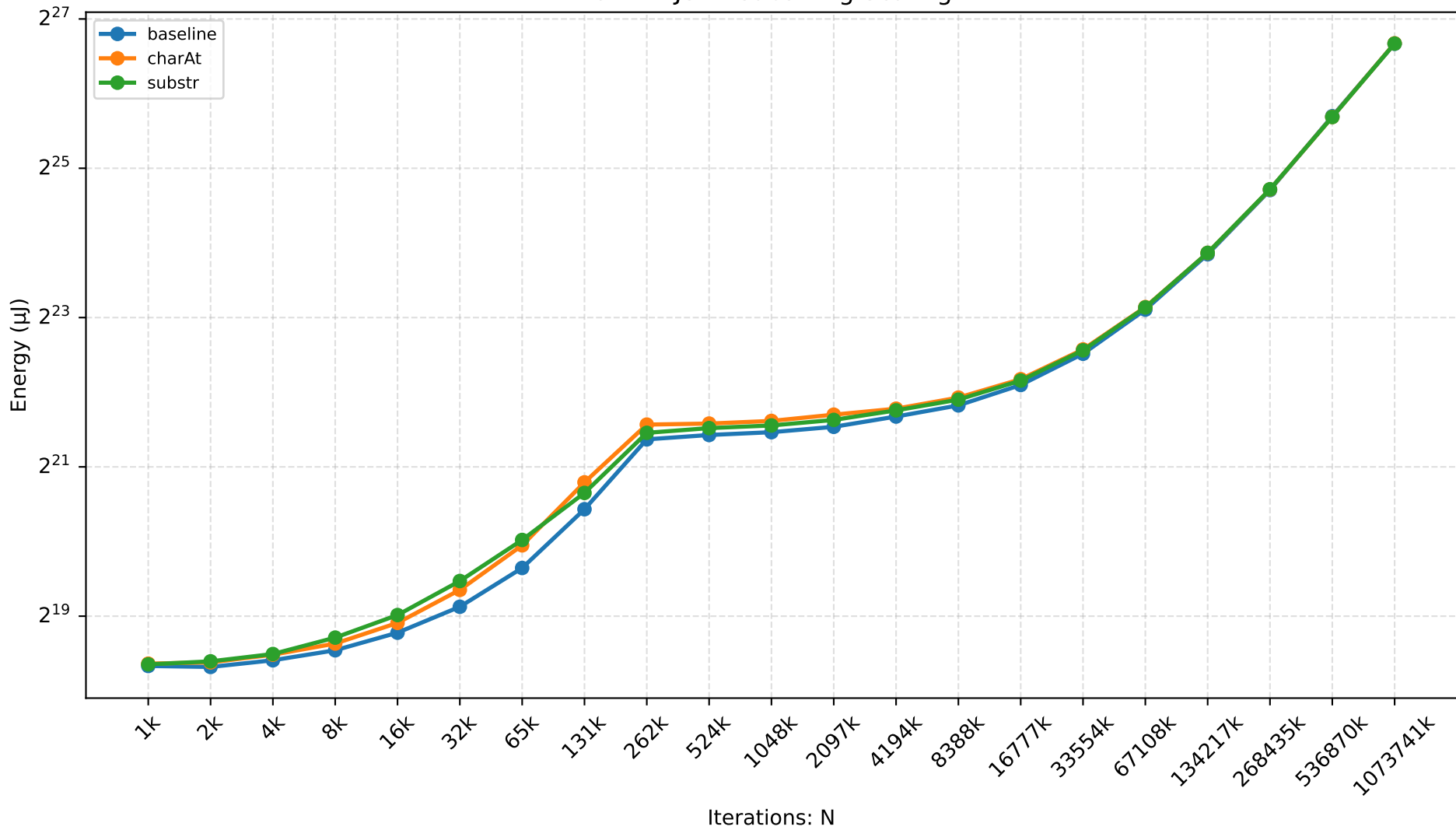
GRAALJS — substring Scaling
