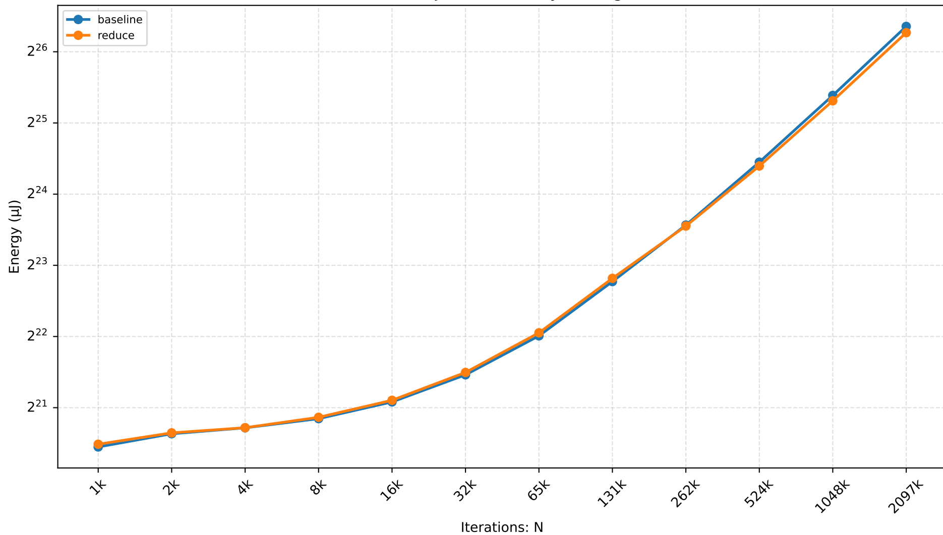
GRAALJS — sum-array Scaling
