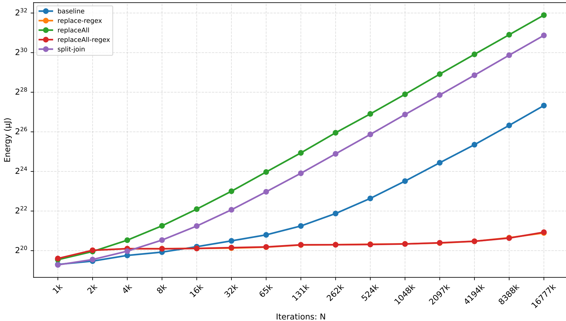
JSC — replace-loop Scaling
