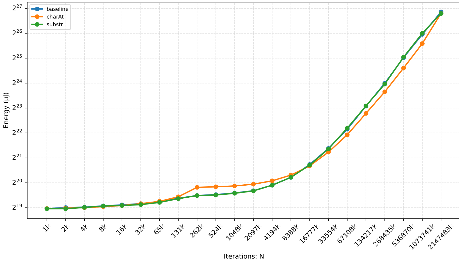
JSC — substring Scaling
