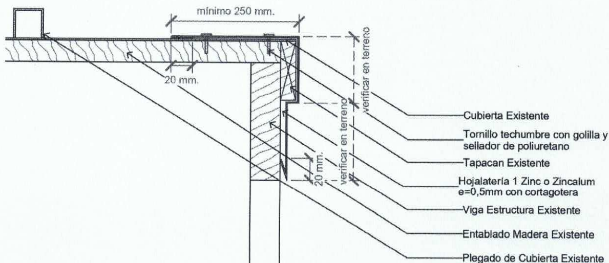
Corte Detalle Hojalaterías alero lateral oriente.
