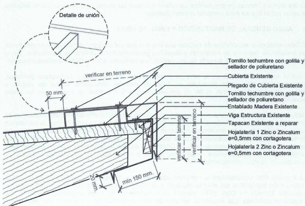
Corte Detalle Hojalaterías alero superior sur.
