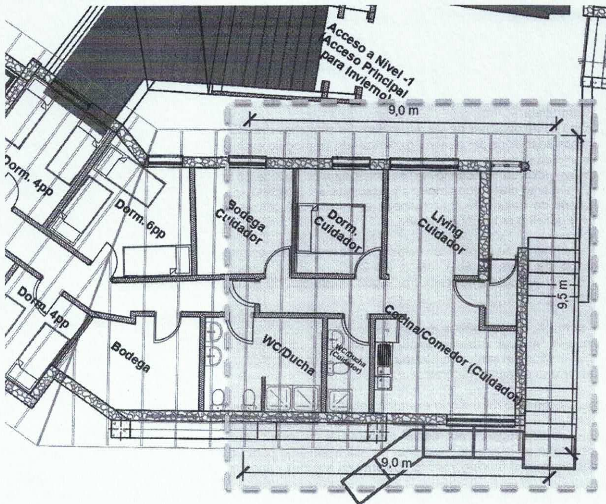
Planta de primer piso de zona a intervenir.
