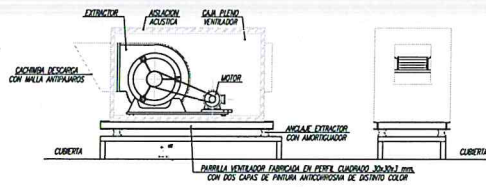
DETALLE MONTAJE EXTRACTOR sin escala
