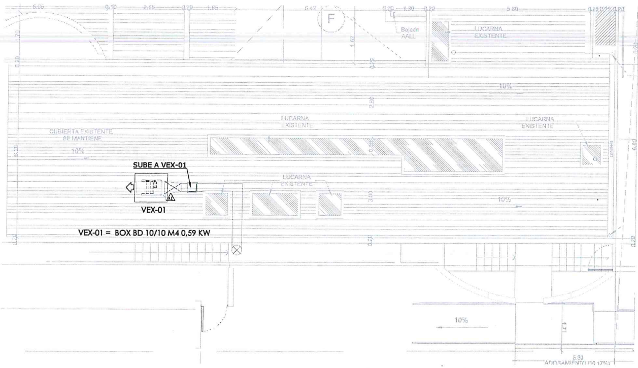
PLANTA DE CUBIERTAS Escala 1:50
