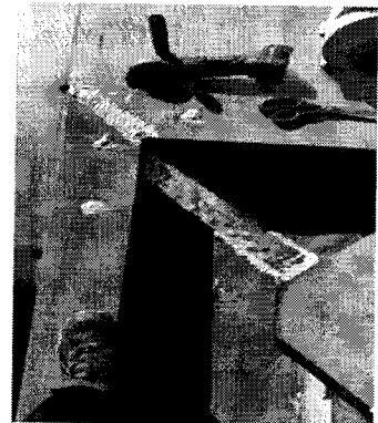
Ilustración 2 Limpieza y aplicación de membrana impermeabilizante aluminizada autoadhesiva.
