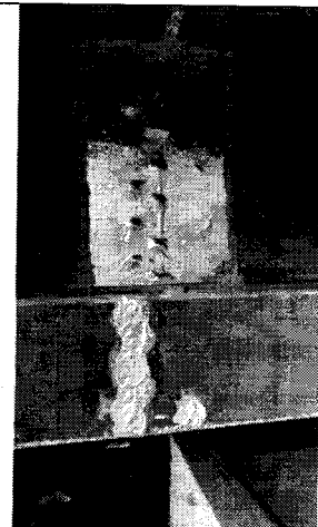
Ilustración 3 Aplicación de sellante de poliuretano para exterior.
