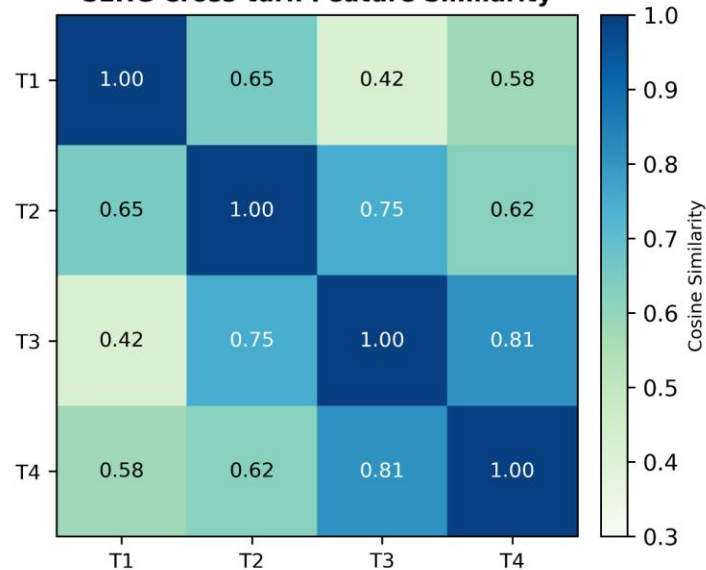
SEHG Cross-turn Feature Similarity
