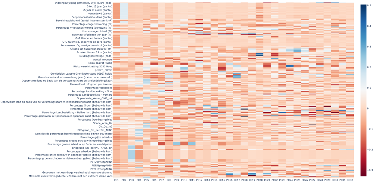
PCA Loadings Heatmap
