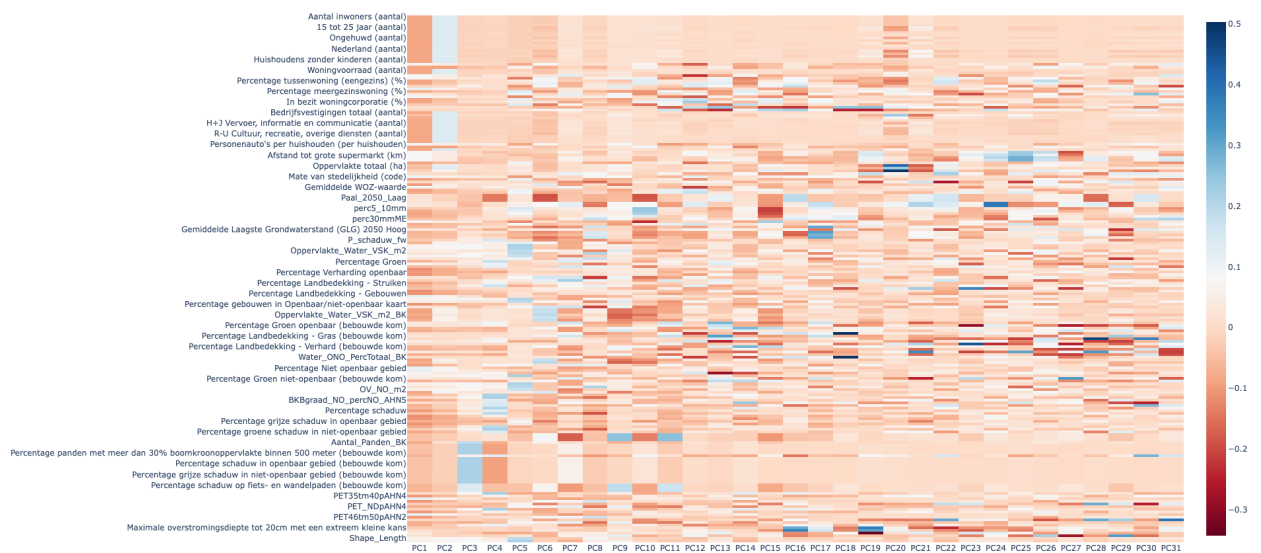
PCA Loadings Heatmap
