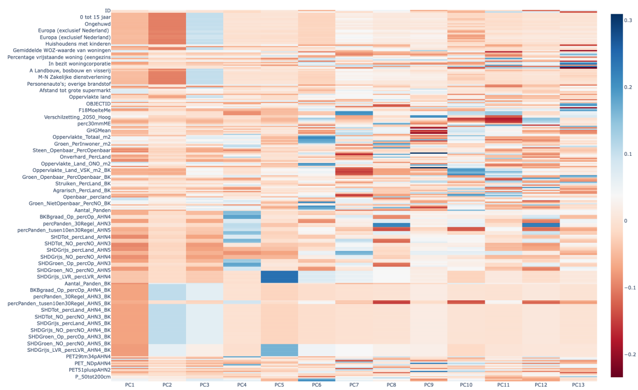
PCA Loadings Heatmap
