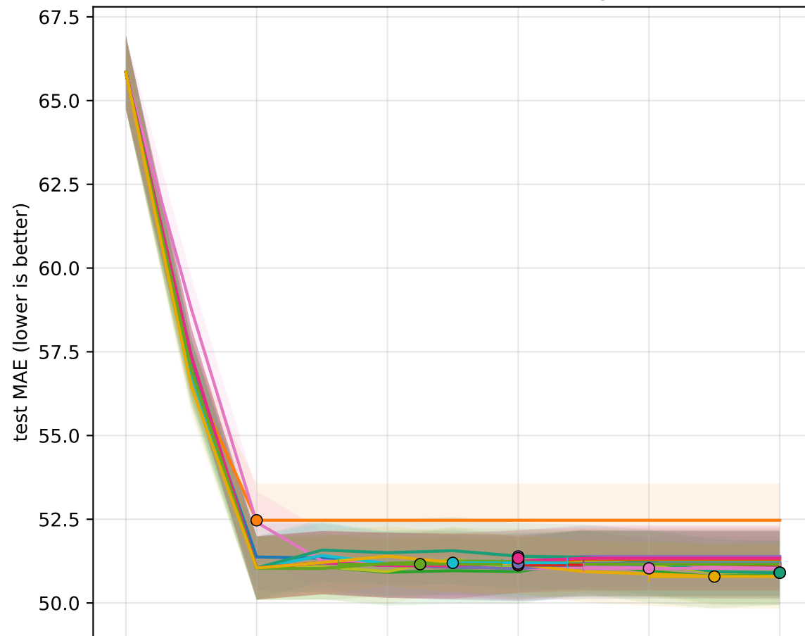
diabetes - GradientBoosting
