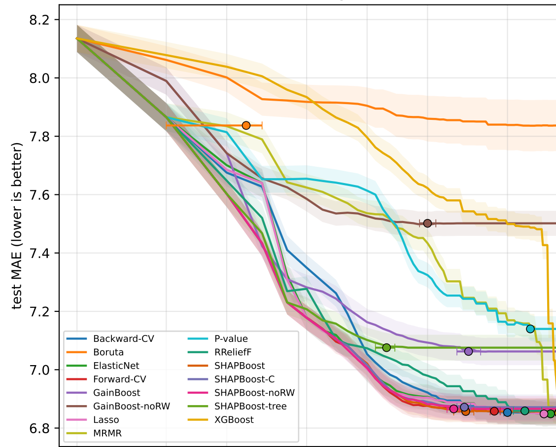
msd - LinearRegression
