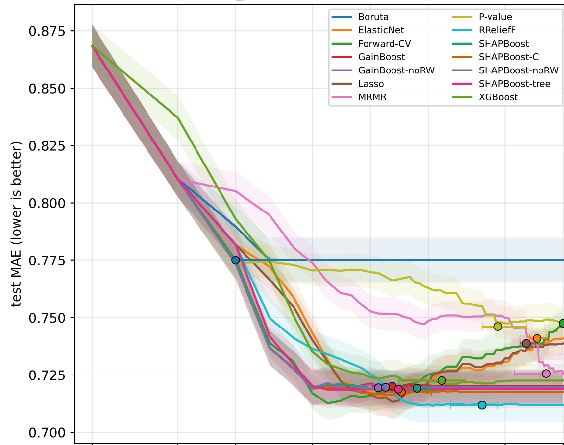
metabarc_regression - LinearRegression
