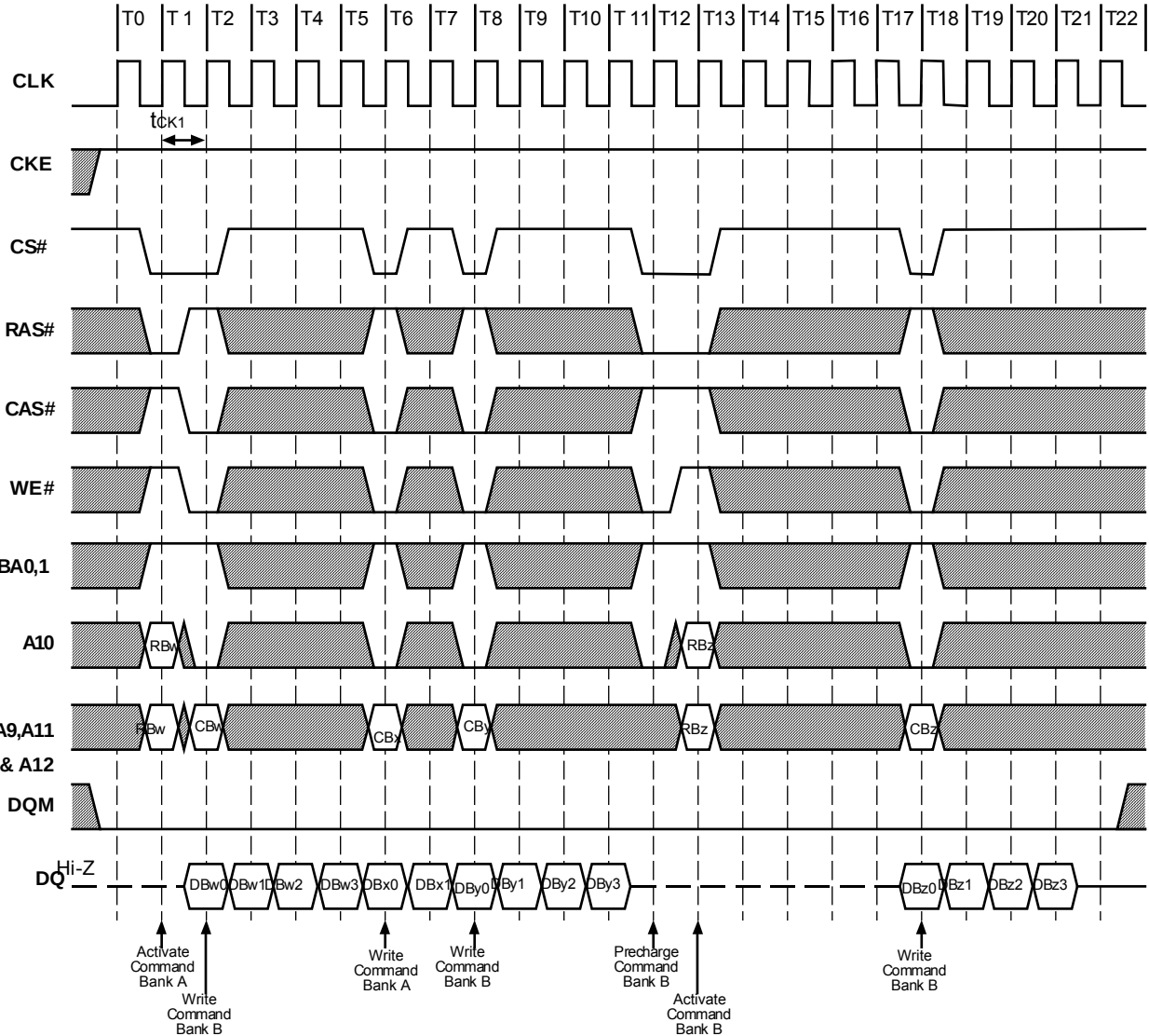
(Burst Length=4, CAS# Latency=1)
