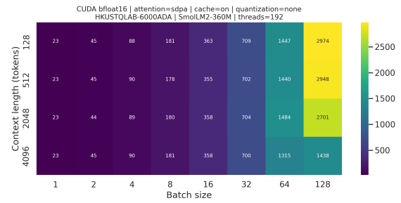
(b) RTX 6000 Ada BF16, batches 1–128
