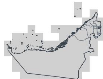
SON 2026 — échéance 1 mois hors saison
