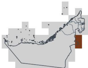
JAS 2026 — en saison hors saison
