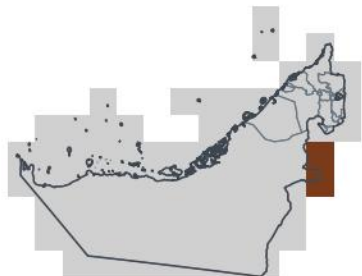
JJA 2026 — en saison hors saison
