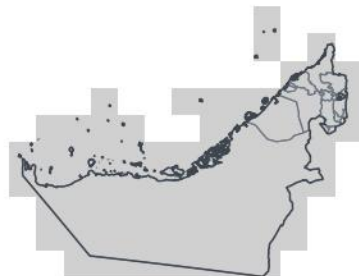
ASO 2026 — en saison hors saison
