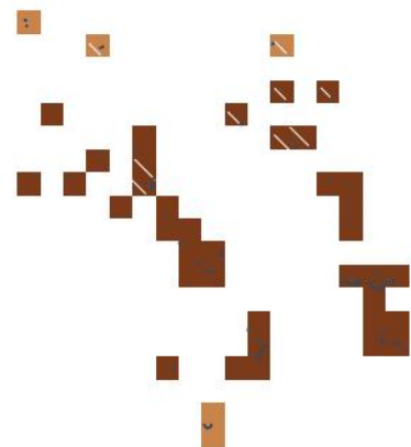
NDJ 2026/27 — échéance 3 mois 1-sur-46 sec · 0e centile
