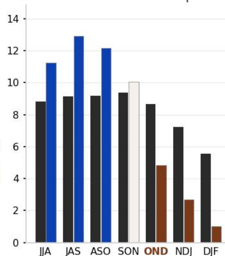
Précipitations moyennes du pays (mm/jour)
