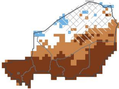
JAS 2026 — en saison 1-sur-15 sec · 4e centile
