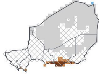
SON 2026 — échéance 1 mois 1-sur-5 sec · 18e centile
