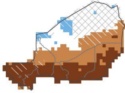
ASO 2026 — en saison 1-sur-12 sec · 7e centile
