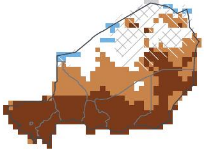
JJA 2026 — en saison 1-sur-23 sec · 2e centile
