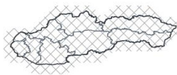
NDJ 2026/27 — échéance 3 mois 1-sur-23 humide · 98e centile
