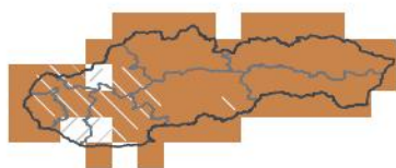
JAS 2026 — en saison 1-sur-4 sec · 22e centile
