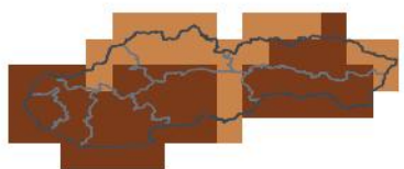
JJA 2026 — en saison 1-sur-15 sec · 4e centile
