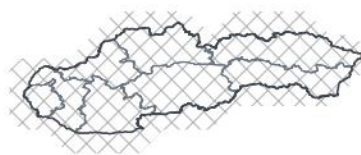
DJF 2026/27 — échéance 4 mois 1-sur-46 humide · 100e centile
