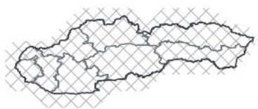
OND 2026 — échéance 2 mois 1-sur-15 humide · 96e centile
